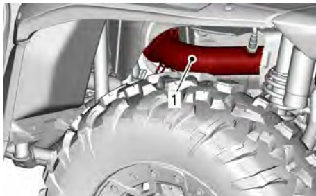
1. Takapakoputki
