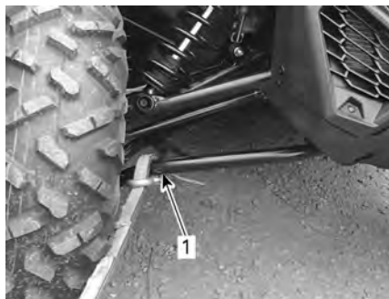
1. Etujousituksien alatukivarsi
