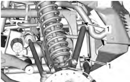
TYYPILLINEN – ETUJOUSITUS
