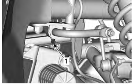
TYPISCH - VOORAAN - STABILISATIESTANG
