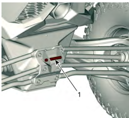
1. Sleephaak achter
