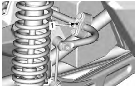
TYPISCH - ACHTERAAN - STABILISATIESTANG
