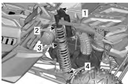
典型示例 - 带回弹阻尼 - 后悬架
