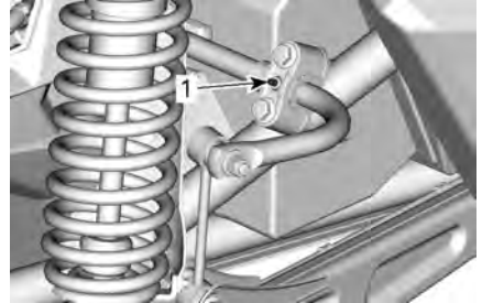
TYPIQUE - BARRE STABILISATRICE ARRIÈRE
