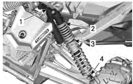
TYPIQUE - AVEC AMORTISSEMENT DE REBOND - SUSPENSION AVANT
