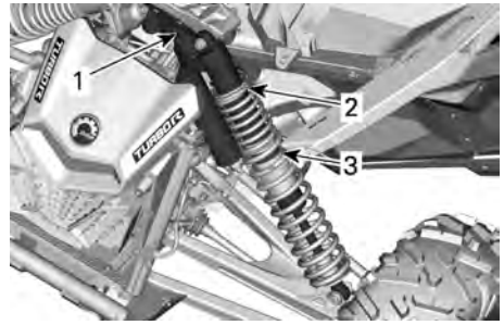
TYPIQUE - SANS AMORTISSEMENT DE REBOND - SUSPENSION AVANT
