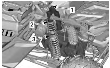
TYPIQUE - SANS AMORTISSEMENT DE REBOND - SUSPENSION ARRIÈRE
