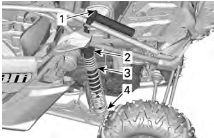
TYPIQUE - AVEC AMORTISSEMENT DE REBOND ET RÉSERVOIR DÉPORTÉ - SUSPENSION ARRIÈRE
