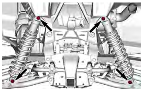
TYPIQUE — FIXATIONS D'AMORTISSEUR ARRIÈRE
