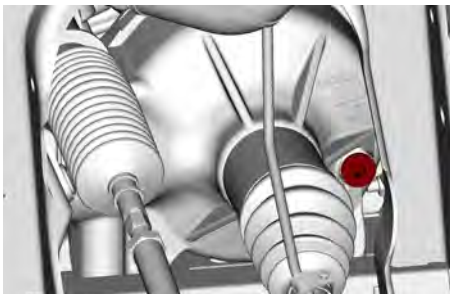
FRÄMRE DIFFERENTIAL (UTAN STÅLLDON)
