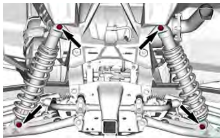
TYPBILD — BAKRE STÖTDÄMPARNAS FÄSTELEMENT
