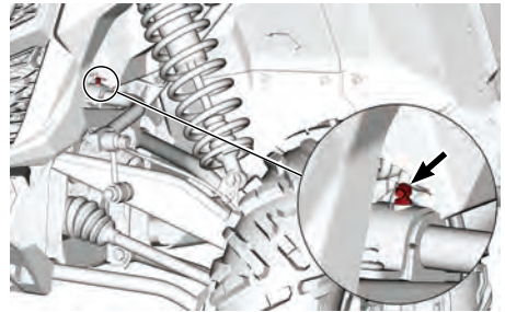
TYPBILD — KRÄNGNINGSHÄMMARE
