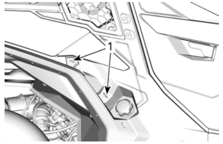
1. Kvartsvarvsfästen
