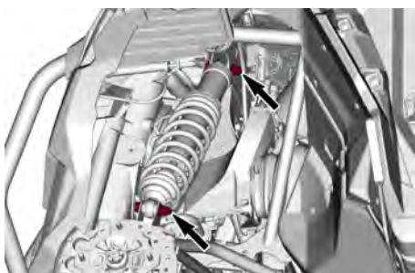
TYPIQUE — FIXATIONS D'AMORTISSEUR AVANT
