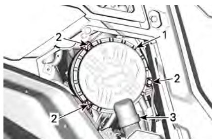
TYPIQUE - CÔTÉ DROIT DU VÉHICULE, SOUS LA BOÎTE DE CHARGEMENT
