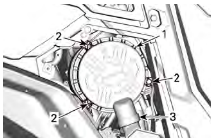
1. Ilmansuodattimen kansi
