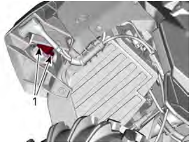
RIKTNINGSVISARENS LAMPFATTNING
