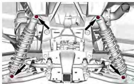
TIPIQUE — FIXATIONS D'AMORTISSEUR ARRIÈRE
