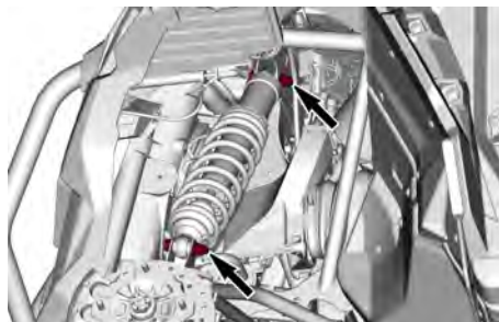
TIPIQUE — FIXATIONS D'AMORTISSEUR AVANT
