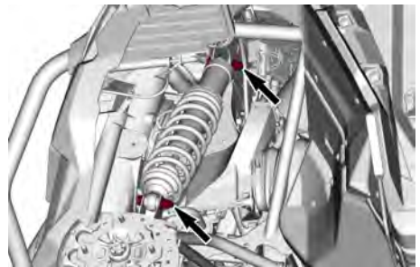
TYPISCH — BEVESTIGINGEN SCHOK-DEMPEER VOOR
