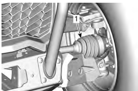
TYPBILD — FRAMHJULSIDA
