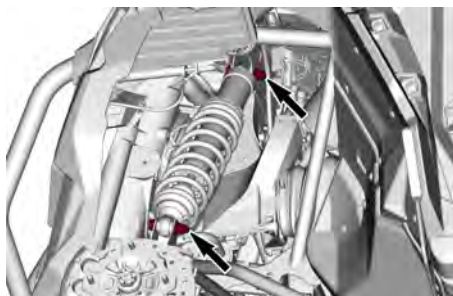
TYPISK - STØTDEMPERFESTER FORAN
