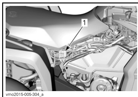
1. Sikringsholder bak
