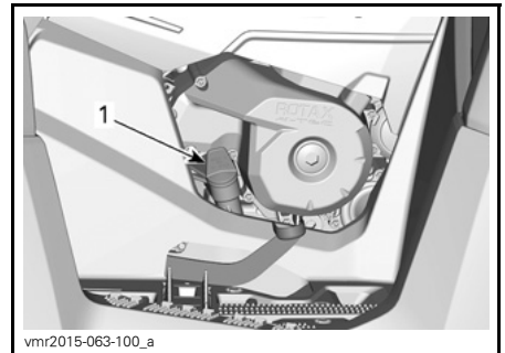
500-MODELL – HØYRE SIDE AV MOTOREN 1. Peilestav
