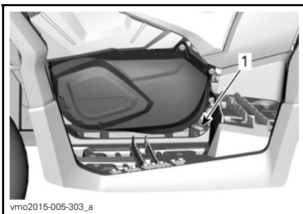
vmo2015-005-303_a 500-MODELLER 1. CVT-avtappingsplugg
