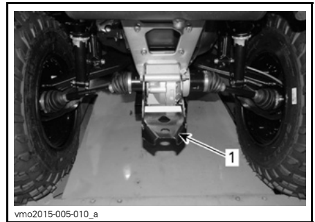
1. Bergingskrok
