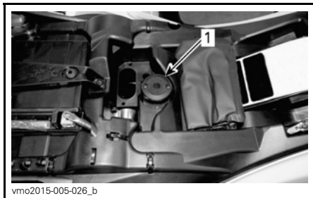
1. Bremsevæskebeholder for bremser bak
