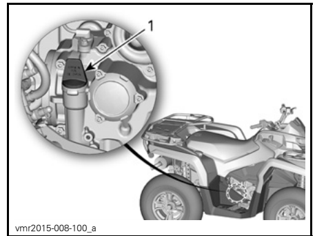
450-MODELL – HØYRE SIDE AV MOTOREN 1. Peilestav
