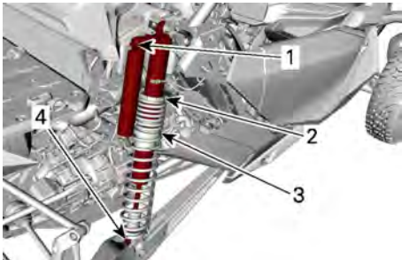
TYPIQUE - SUSPENSION ARRIÈRE
