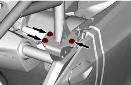
DISPOSITIVI DI FISSAGGIO CENTRALI INFERIORI – CONFIGURAZIONE TIPICA
