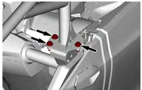
FIXADORES CENTRAIS INFERIORES – TÍPICO
