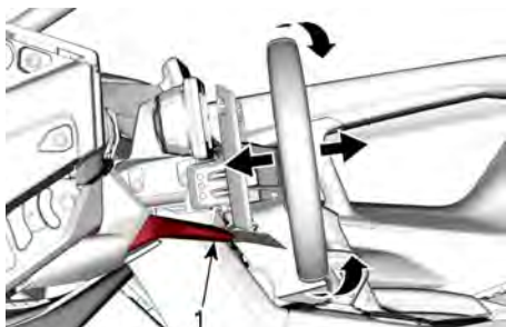
MOVIMENTOS DE INCLINAÇÃO E TELESCÓPICOS
