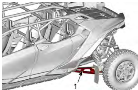
1. Länkmarm
