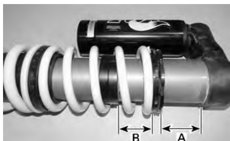
SITUAZIONE TIPICA - REGOLAZIONE CROSSOVER - AMMORTIZZATORE POSTERIORE
