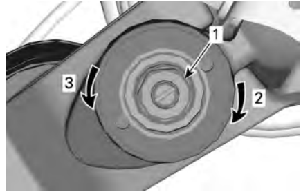
COMPRESSIEDEMPING BIJ HOGE SNELHEID (GEBRUIK EEN SLEUTEL VAN 17 MM)
