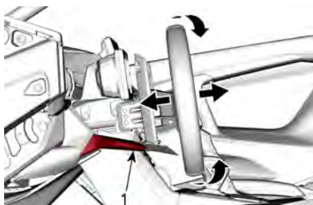
KANTELBEWEGINGEN EN TELESCOPI- SCHE BEWEGINGEN
