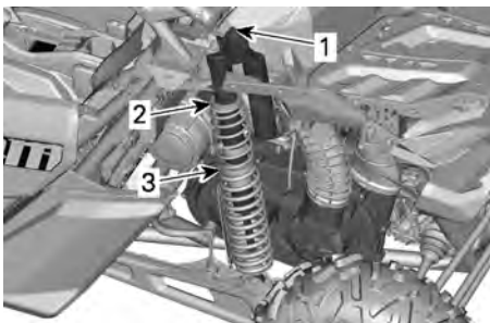
TYPIQUE - SANS AMORTISSEMENT DE REBOND - SUSPENSION ARRIÈRE
