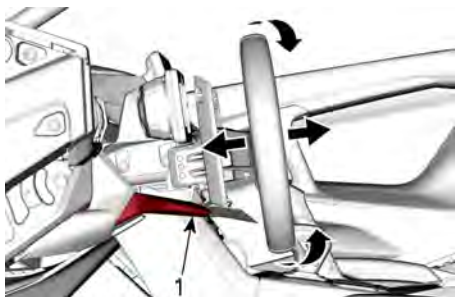
KANTELENGEBEWEGINGEN EN TELESCOPI- SCHE BEWEGINGEN
