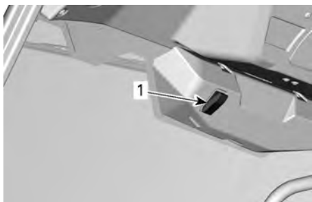
1. Commutateur d'essuie-glace
