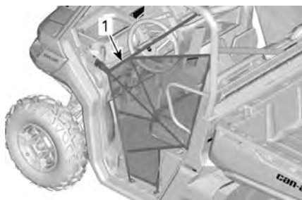
1. 侧边安全网
