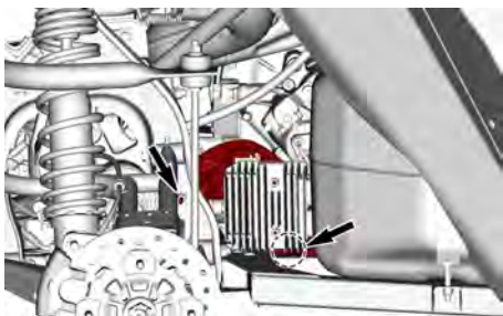
电压/调节器支架紧固件位置
