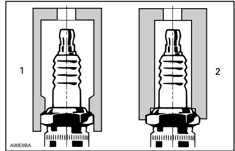
1. Korrekt gänga
