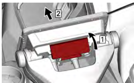
Trinn 1. Løft tappen
