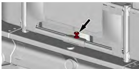
COUVERCLE DU COMPARTIMENT DE RANGEMENT DE L'ANCRE
