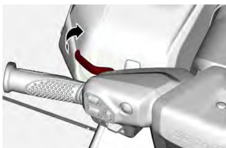
LEVIER iBR RELÂCHÉ
