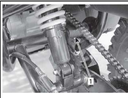
1. Aandrijfkettingrol
