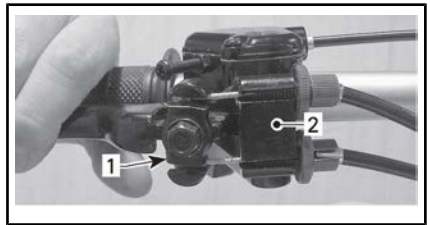
1. Kabellink
