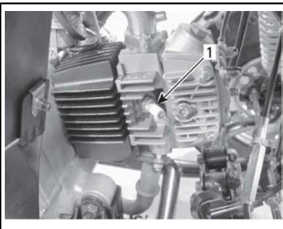
1. Ontstekingsbougie
