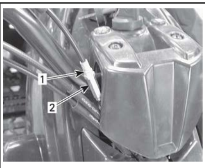
1. Borgmoer 2. Afstelschroef
