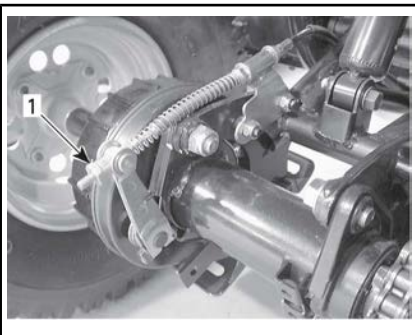
1. Regelaar remkabel
