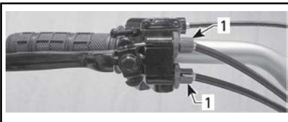
1. Schroeven voor aanpassing op de hendel
