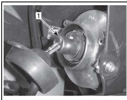
DUW EN DRAAI DE LAMPHOUDER LINKSOM
