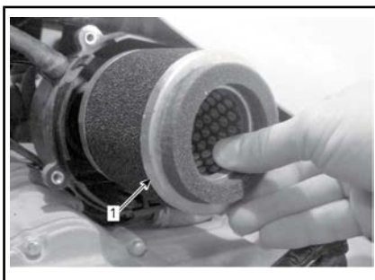
1. Luchtfilter
