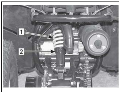
DS 90: ACHTEROPHANGING
