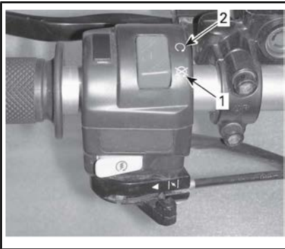
TYPISCH - MOTORSTOPSCHAKELAAR
