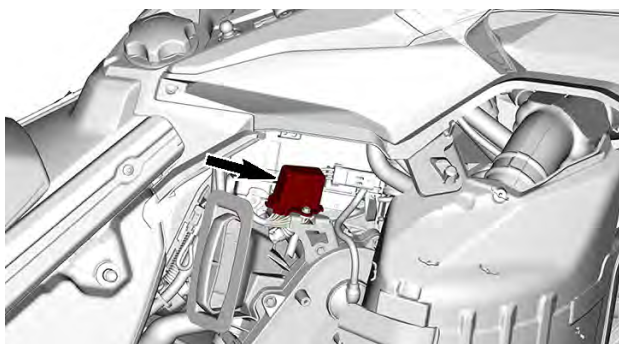
SCATOLA FUSIBILI 1 (FB1) – MOTORI E-TEC 400 MM (16 IN)
