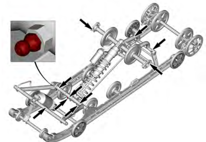
EASY RIDE+ FS UTAN SNABBJUSTERANDE BAKSTATIV
