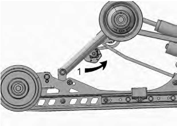
TYPBILD – HÖGER SIDA
