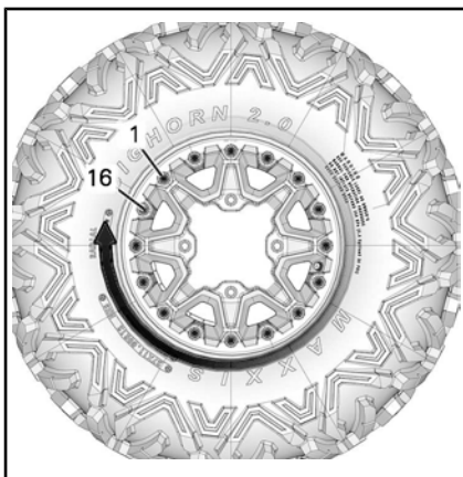
代表例 - 最後の締め付け順序
