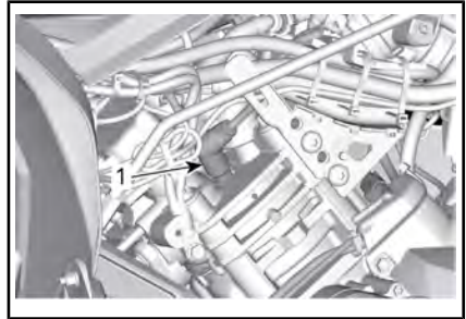
左側 — フロントシリンダー 1. スパークプラグ
