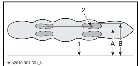
TYPISK STRÅLKASTARREFLEKTION PÅ TESTYTAN
