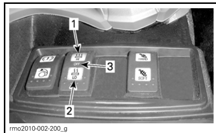
1. HI (högvärmeläge) 2. LO (lågvärmeläge) 3. AV (mittlege)
