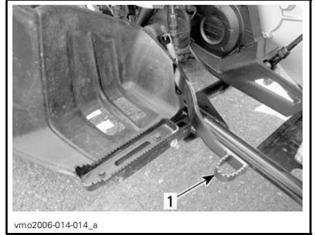
1. Pédale de frein arrière
