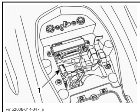
1. Porte-fusible
