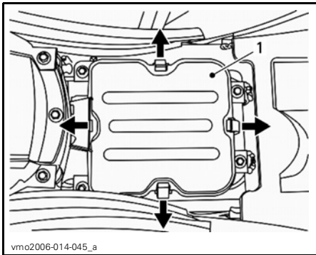
1. Couvercle du boîtier de filtre à air
