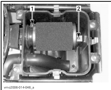
1. Collier 2. Vis de fixation
