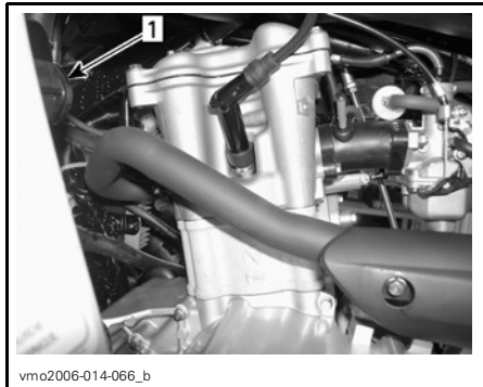
CÔTÉ GAUCHE DU MOTEUR 1. Soupape d'injection d'air
