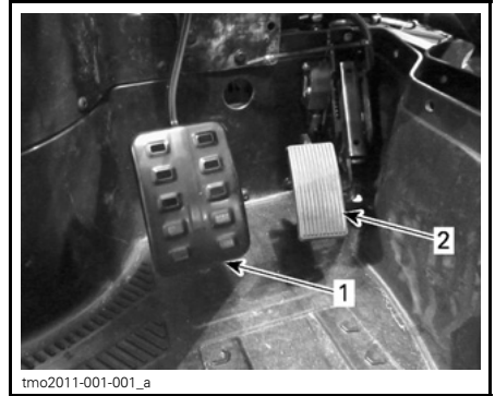
1. Jarrupoljin 2. Kaasupoljin
