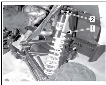
SUSPENSÃO TRASEIRA — MODELOS COM DPS
