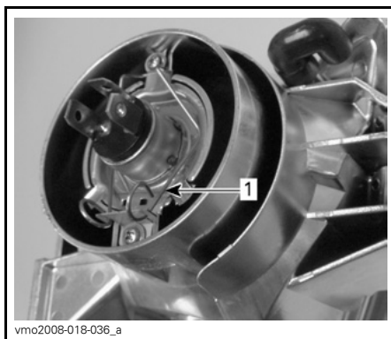
TYPISCH 1. Houderclip
