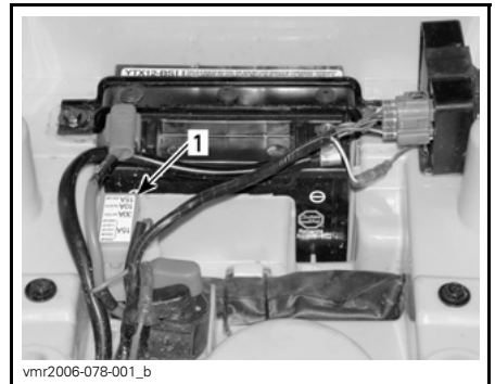
1. Zekeringhouder
