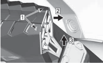
1. CVT-Luftfilter
