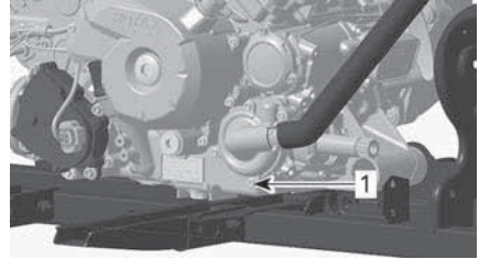
1. Kühlmittelablassschraube
