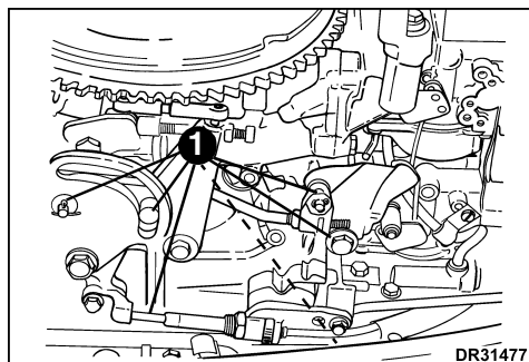
1. Tringlerie d'accélération 2. Tringlerie de commande de sens de marche
