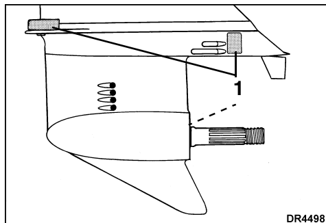
1. Anodes anticorrosion
