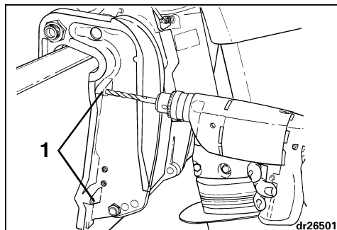
1. Perçage de trous dans le tableau arrière
