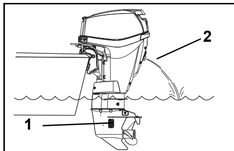
1. Crépines de prises d'eau 2. Indicateur de pompe à eau
