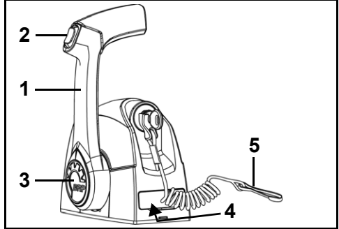
Commande à levier unique montée sur l'habitacle 006446
