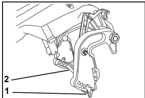
1. Dispositif de retenue de l'axe de relevage 007025 2. Axe de relevage
