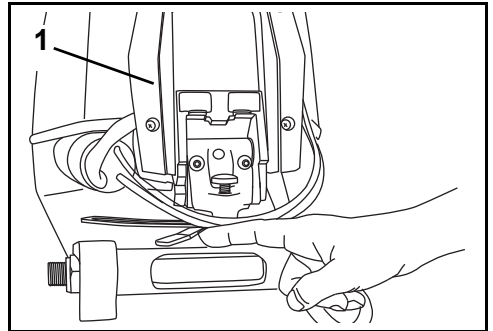
1. Levier de friction de la direction 007042
